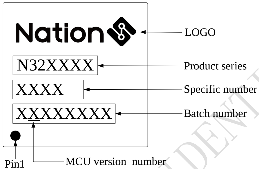
图 5-7 LQFP48/LQFP64/LQFP100 丝印说明
