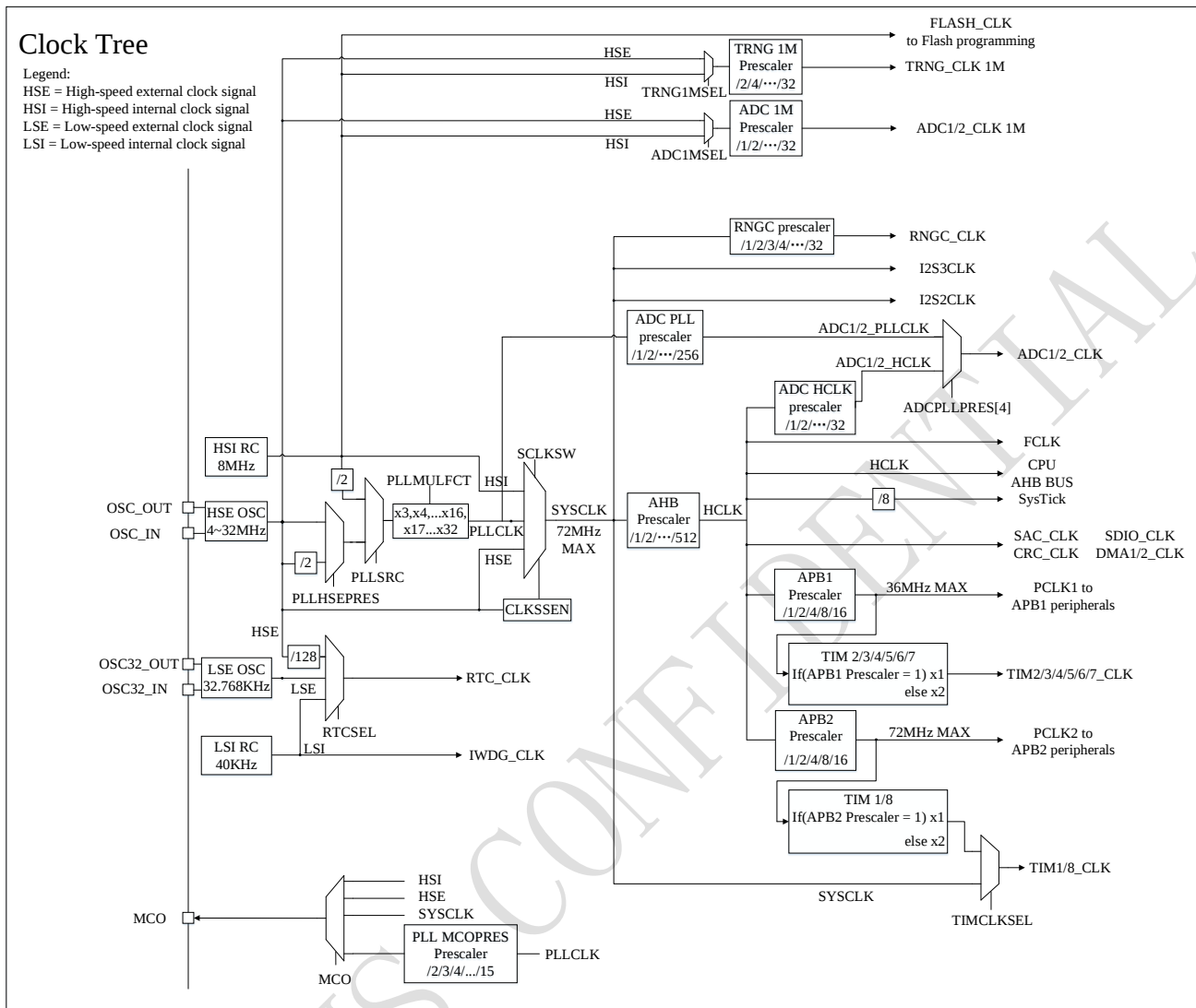
图 2-2 时钟树
