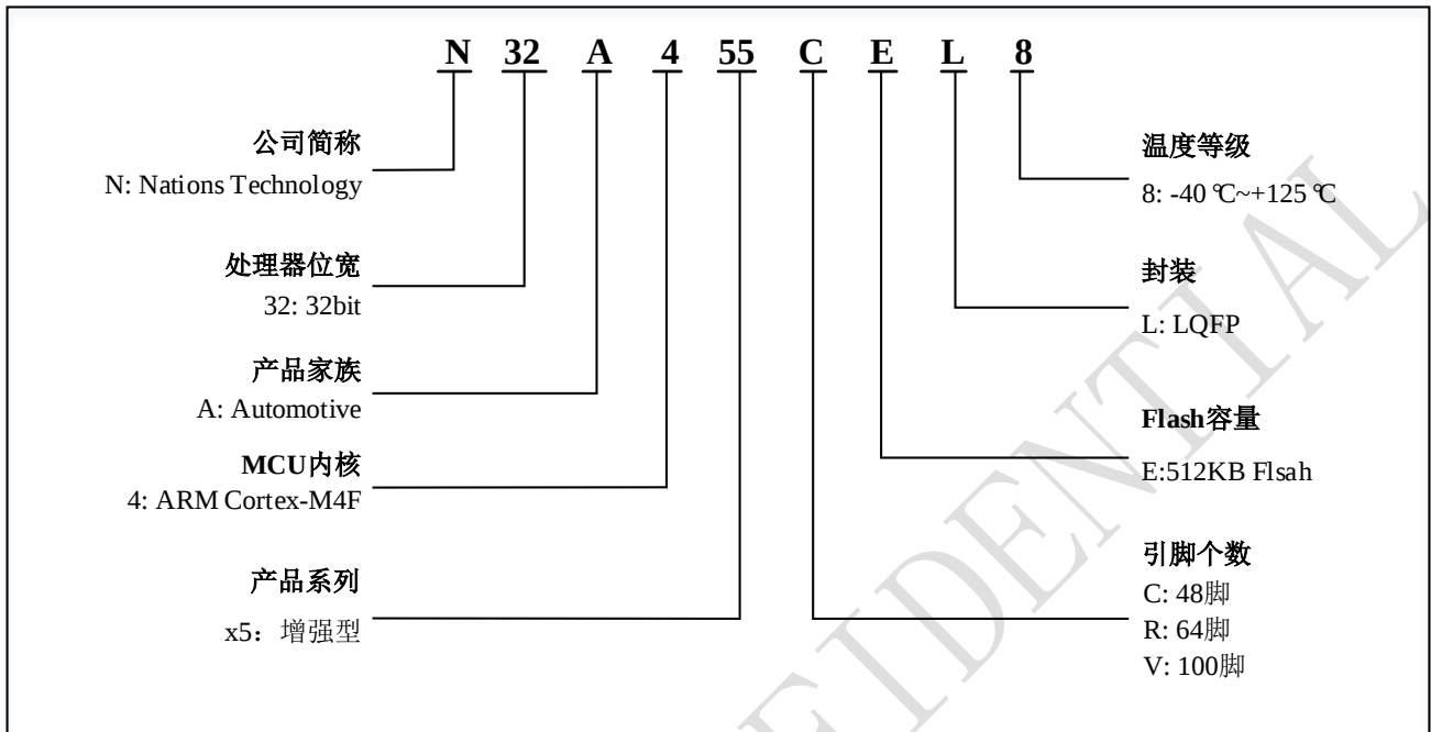
图 6-1 N32A455系列订货代码信息图示
