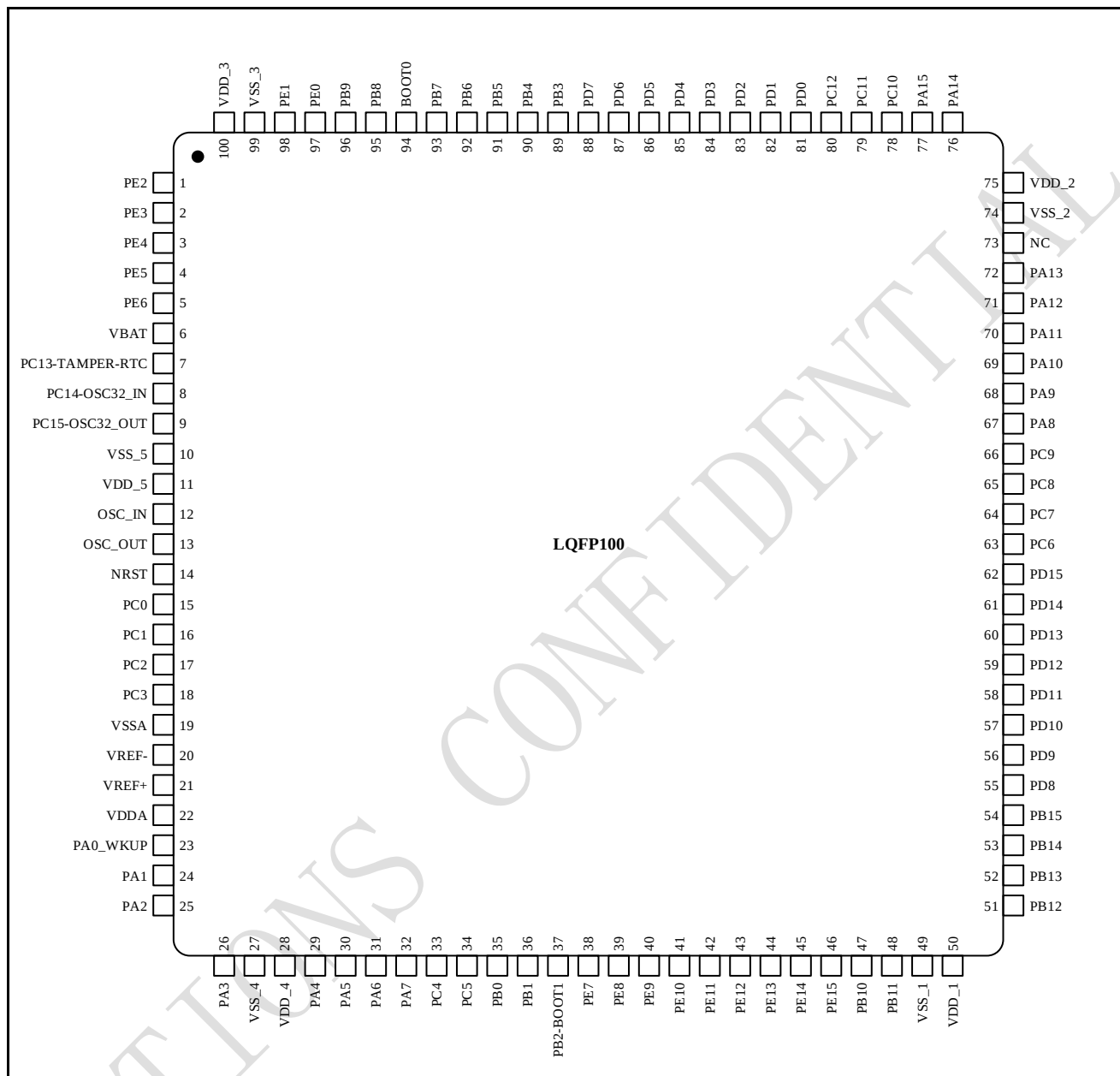
图 3-3 N32A455xxL8系列LQFP100引脚分布
