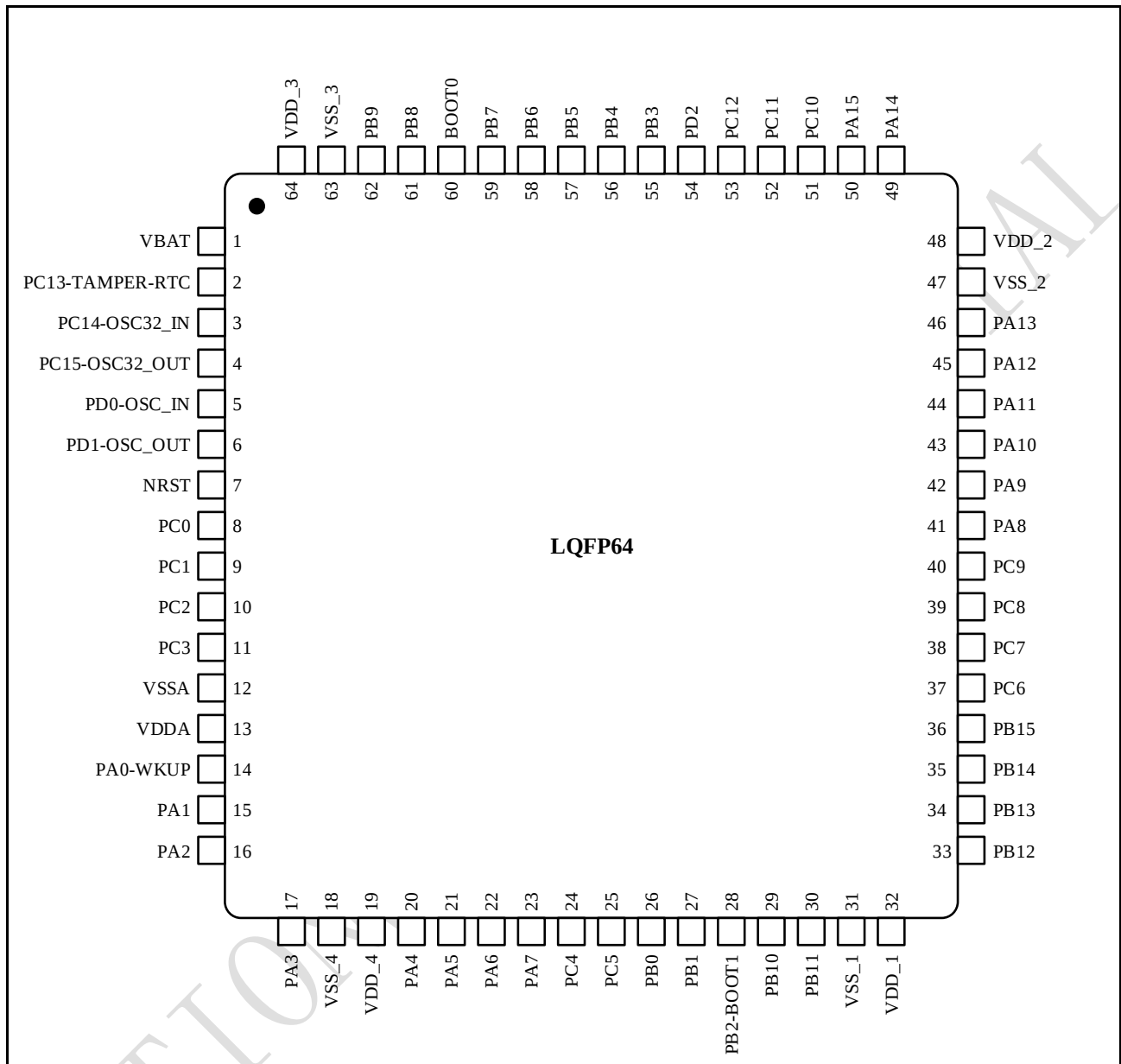
图 3-2 N32A455xxL8系列LQFP64引脚分布
