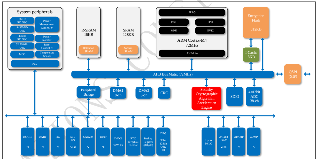
图 1-1 N32A455xxL8系列框图
