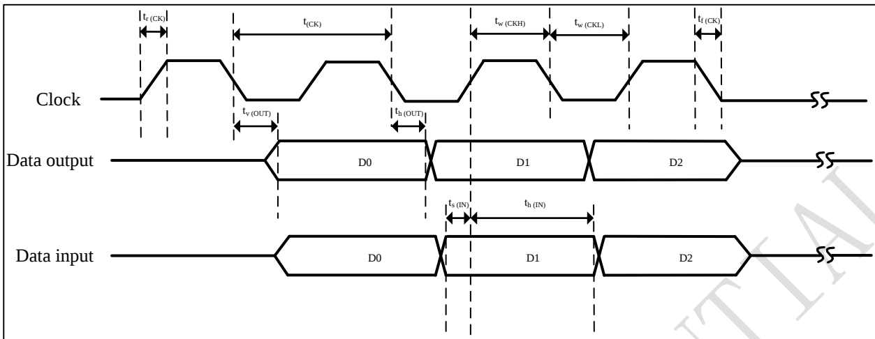
图 4-18 QSPI在SDR模式下的时序
