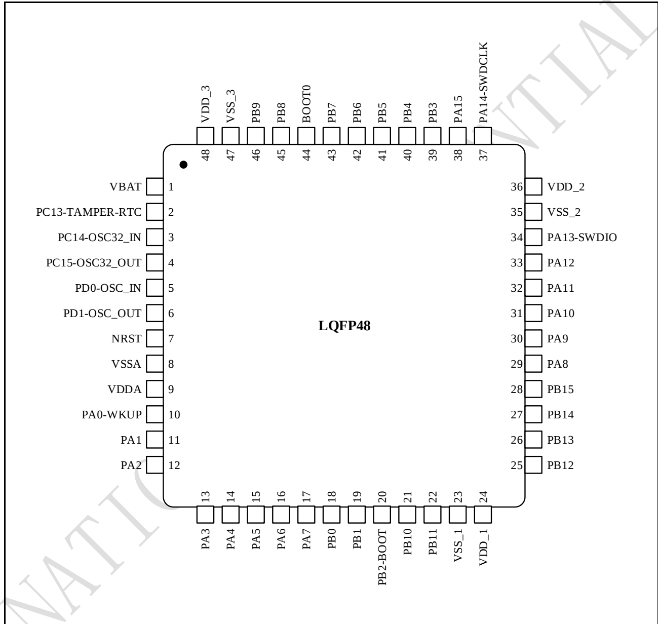
图 3-1 N32A455xxL8系列LQFP48引脚分布
